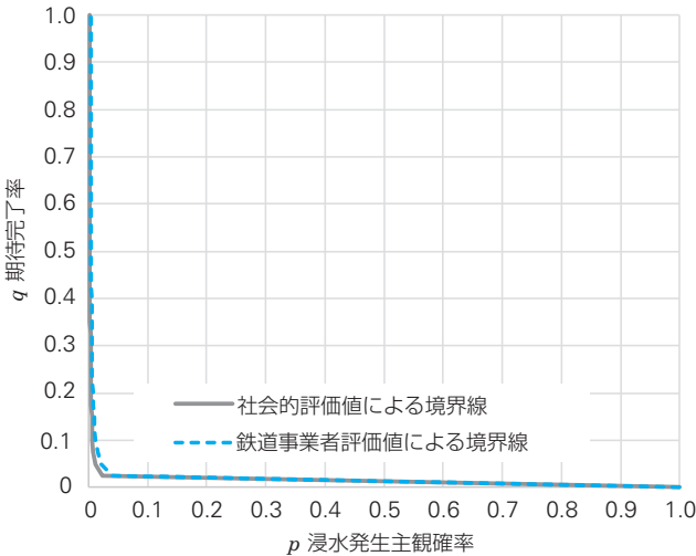
■図—4 東北新幹線那須電車留置線事例の計算結果
