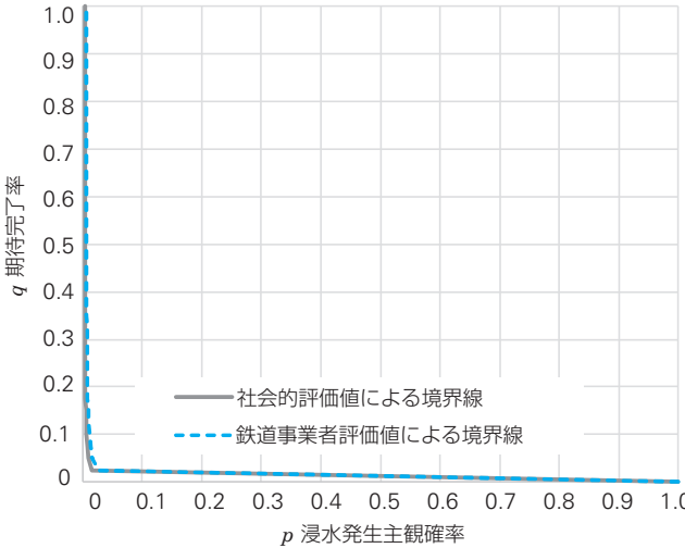
■図—5 北陸新幹線長野車両基地事例の計算結果
